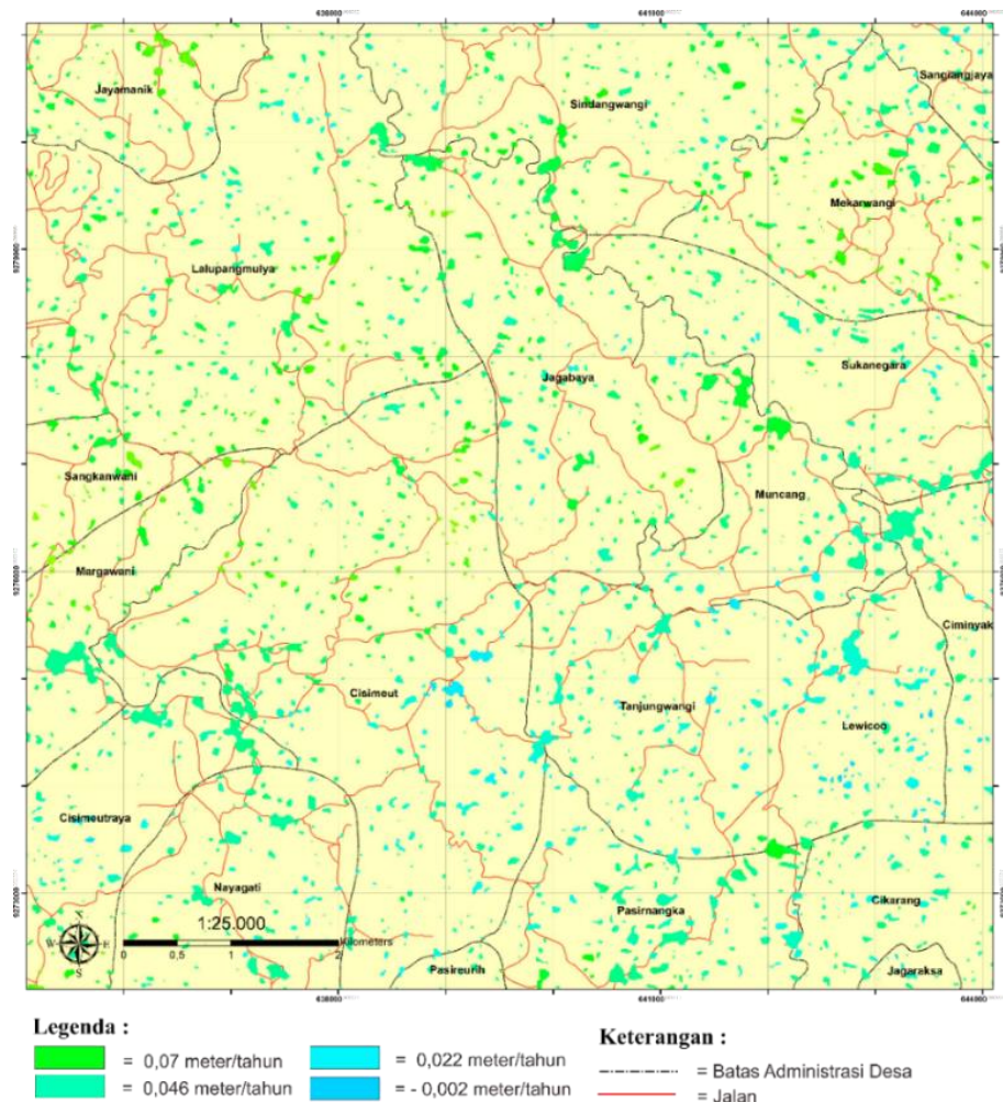
Gambar 5. Peta Perubahan Muka Tanah Tahun 2020
