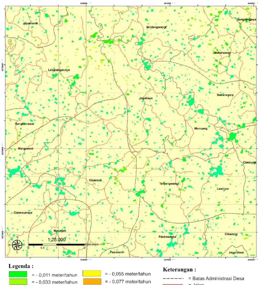
Gambar 6. Peta Perubahan Muka Tanah Tahun 2021
