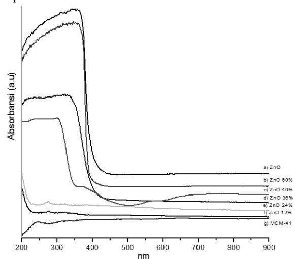
Gambar 4. Spektra DR-UV ZnO/MCM-41 pada berbagai konsentrasi Zn
