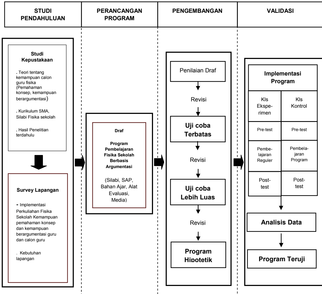
Gambar 2. Desain Penelitian
