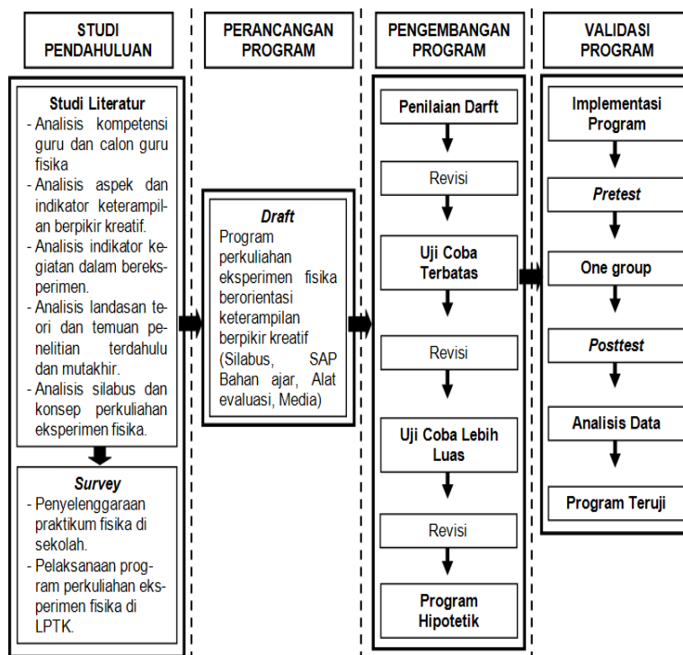
Gambar 1. Desain Penelitian
