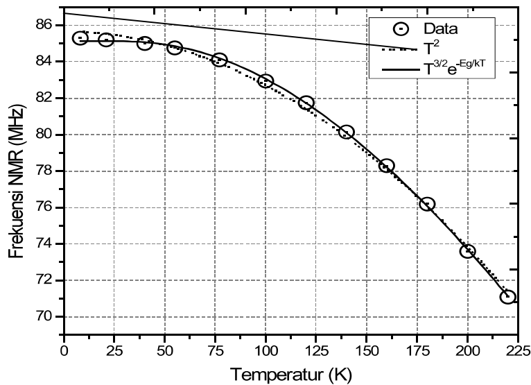
Gambar 6. Hubungan antara frekuensi NMR sampel terhadap temperatur. Lingkaran hitam merupakan data eksperimen dari frekuensi resonansi NMR pada bahan FeF_3 .
