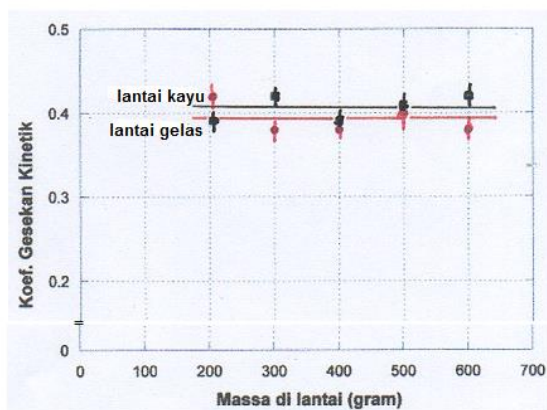
Gambar 5. Koefisien gesekan kinetik sebagai fungsi massa silinder logam (luas penampang alasnya tetap) yang bergerak di lantai gelas dan kayu ketika melakukan GLB.
