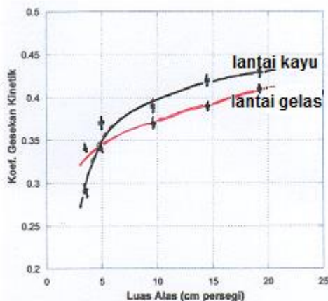
Gambar 4. Koefisien gesekan kinetik sebagai fungsi luas penampang alas silinder logam (massa tetap) yang bergerak di lantai gelas dan kayu ketika melakukan GLB.
