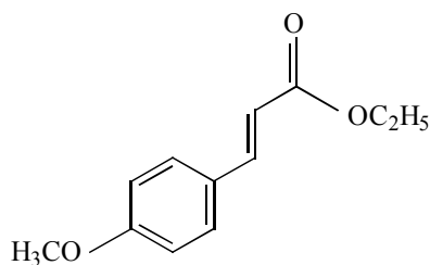
Gambar 1. Etil p-Metoksisinamat
