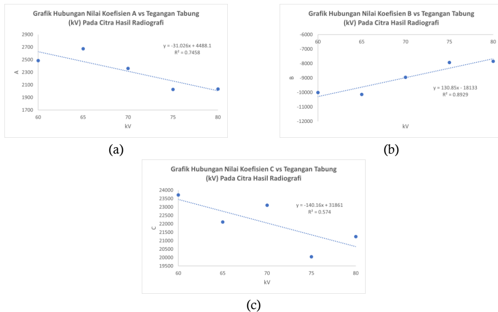
Graph 2. Grafik linear hubungan nilai koefisien dan variasi tegangan tabung (kV) (a) Koefisien A; (b) Koefisien B; (c) Koefisien C
