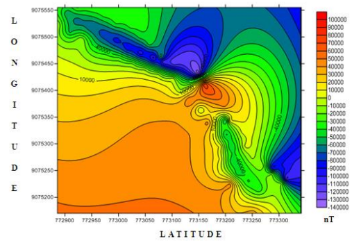
Gambar 6. Pola Kontur hasil Kontinuitas Atas dengan 100 mdatum
