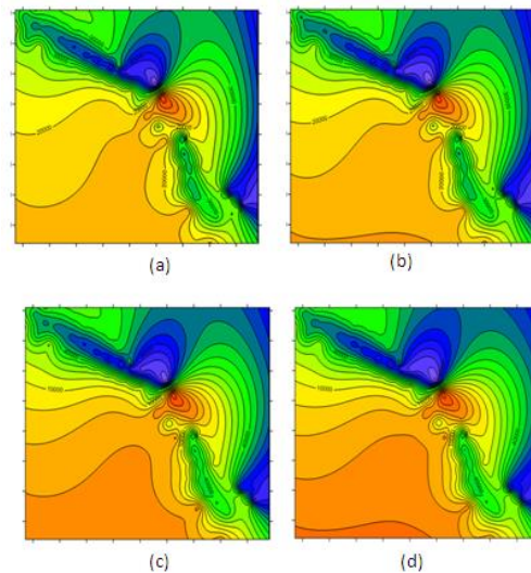
Gambar 7. Pola Kontur hasil Kontinuitas Atas gabungan (a). 70 mdatum, (b). 80 mdatum, (c) 90 mdatum dan (d) 100 mdatum
