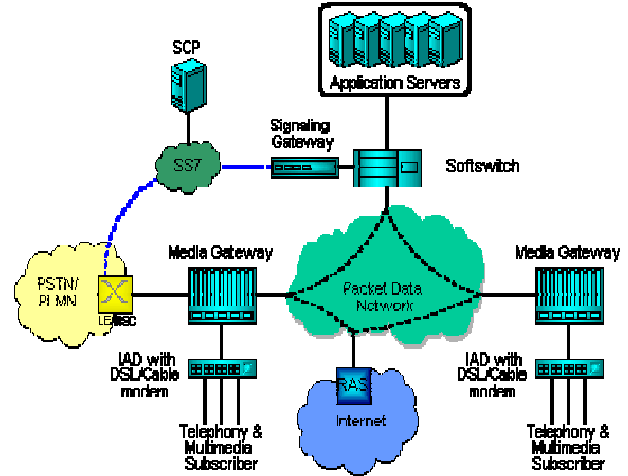
Gambar 2. Arsitektur Jaringan Softswitch
