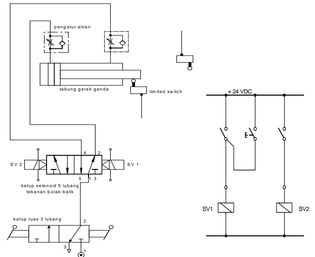
Gambar 9. Diagram Alir
