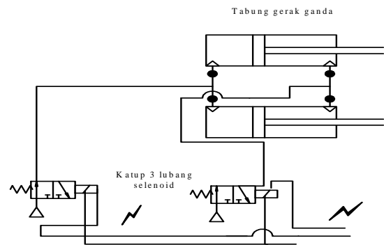
Rancangan 2 dengan 2 katup selenoid 3 lubang & tabung gerak tunggal
