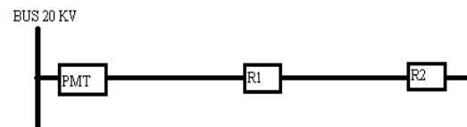
Gambar 7. koordinasi OCR
