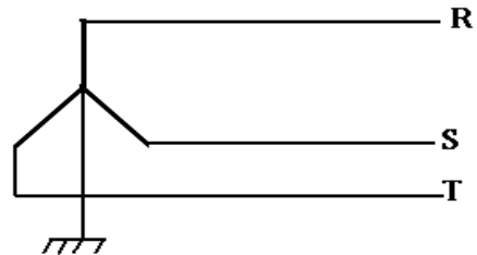
Gambar 2. Diagram sistem pentanahan pola 2
