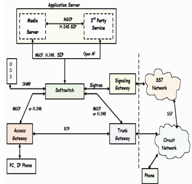
Gambar 6. Protokol-protokol pada Softswitch [Ludfy, 2005]
