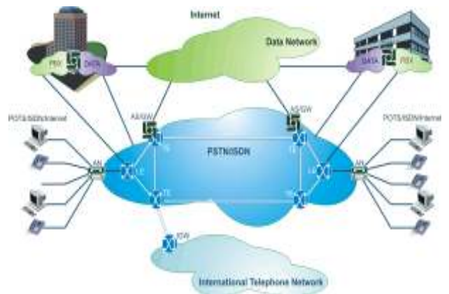
Gambar 2. Jaringan Telekomunikasi Kini [Trans Komunikasi Data, 2005]
