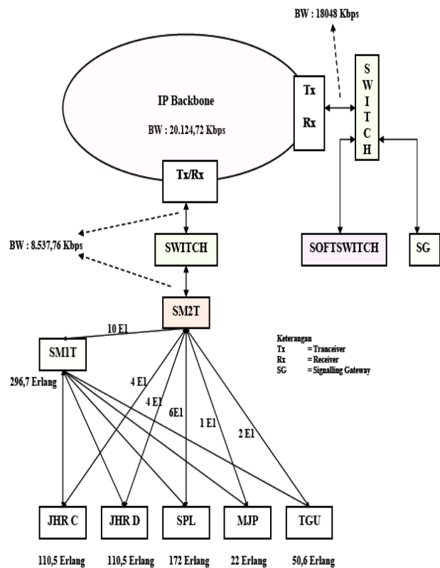
Gambar 10. Konfigurasi Jaringan Terintegrasi Softswitch Semarang
