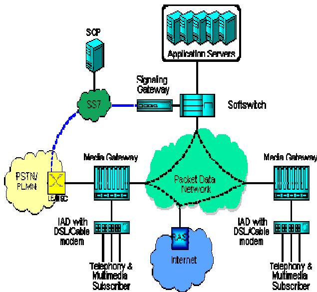
Gambar 5. Arsitektur Jaringan Softswitch [Widodo, 2005]
