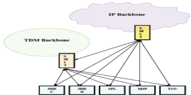
Gambar 9. Topologi Jaringan PSTN dengan Trunk Gateway Softswitch yang terintegrasi [PT. Telkom, 2005]
