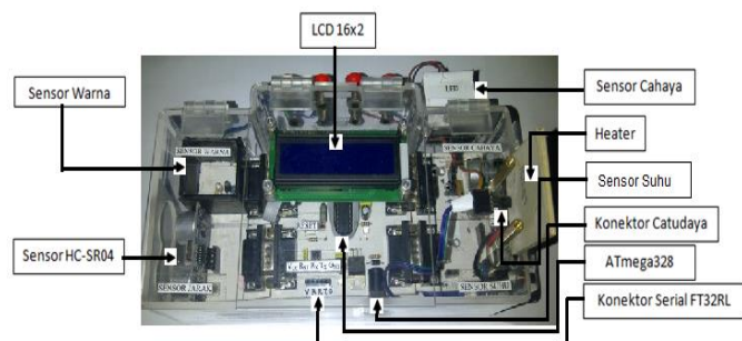
Gambar 8. Trainer Sensor Berbasis Arduino
