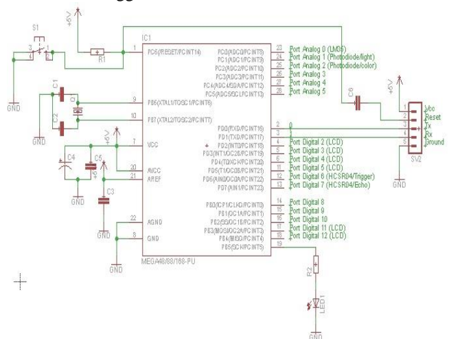
Gambar 1. Rangkaian mainboard
