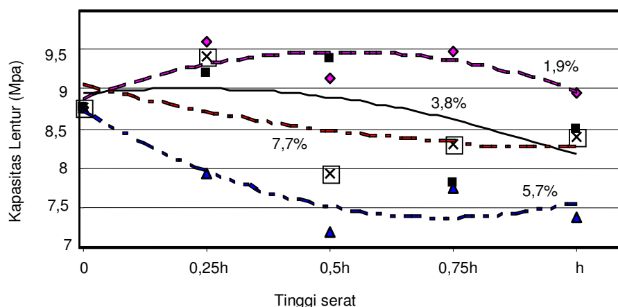
Gambar 8. Pengaruh Konsentrasi Serat terhadap Kapasitas Lentur
