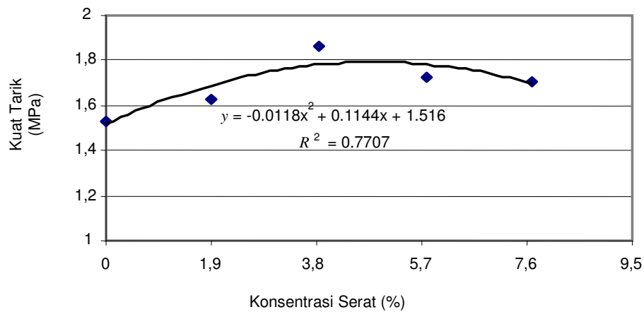
Gambar 5. Hubungan Konsentrasi Serat terhadap Kuat Tarik Beton
