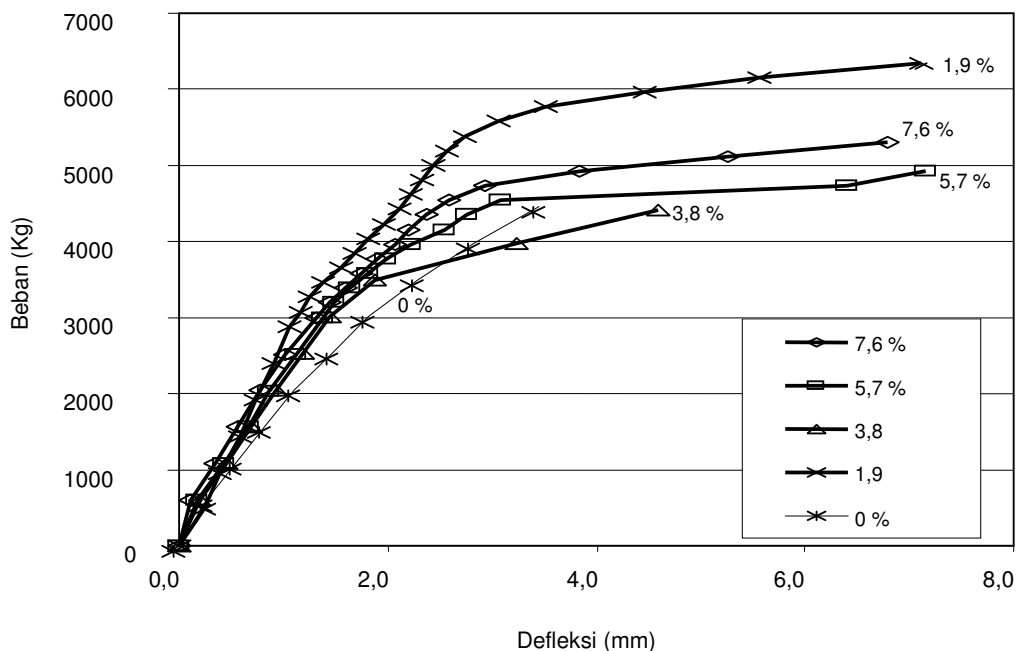
Gambar 7. Hubungan Beban terhadap Defleksi Balok
