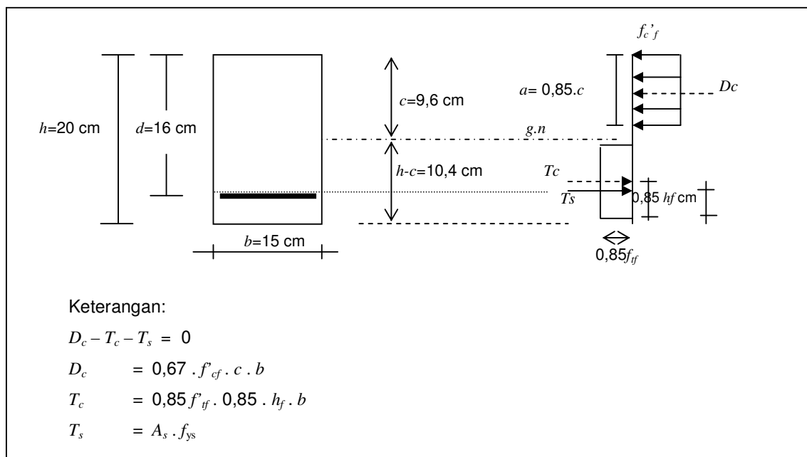
Gambar 3. Analisis Tampang Beton Serat
