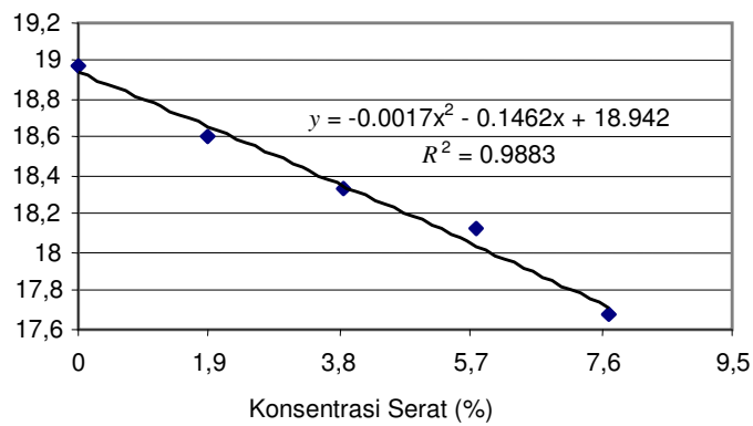
Gambar 4. Hubungan Konsentrasi Serat terhadap Kuat Tarik Beton
