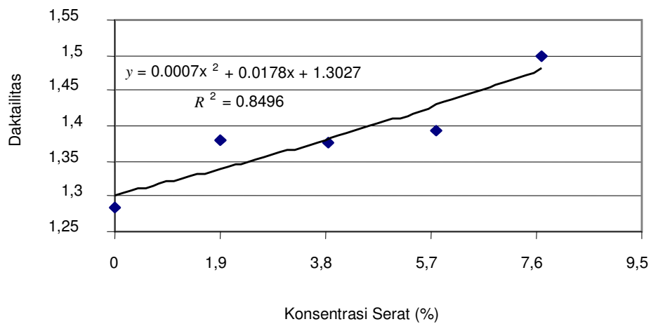
Gambar 6. Hubungan Konsentrasi Serat terhadap Duktailitas
