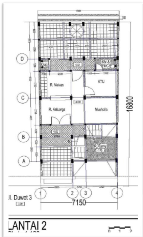
Gambar 2. Denah Lantai Dua Sumber: Dokumentasi, 2014
