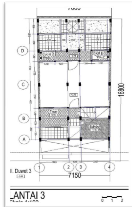
Gambar 3. Denah Lantai Tiga Sumber: Dokumentasi, 2014
