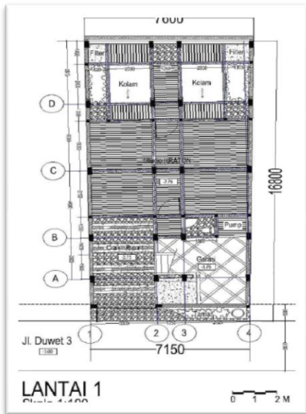
Gambar 1. Denah Lantai Dasar Sumber: Dokumentasi, 2014
