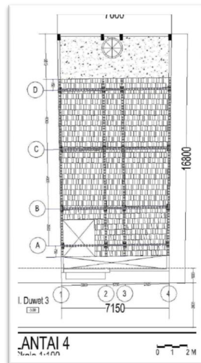
Gambar 4. Denah Lantai Empat Sumber: Dokumentasi, 2014
