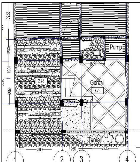
Gambar 6. Letak Toilet Luar Pada Lantai 1 (Satu)
