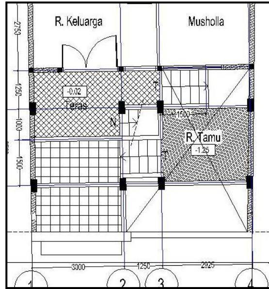
Gambar 7. Letak Ruang Tamu Pada Lantai Mezzanine
