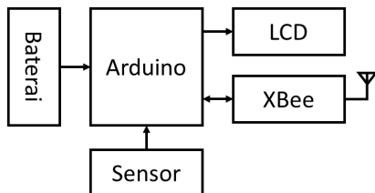
Gambar 2. Diagram blok desain perangkat titik sensor
