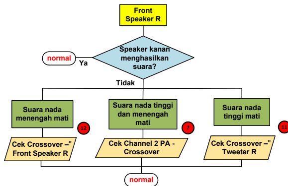
Gambar 13. Flowchart Saklar Trouble 7,11, dan 12
