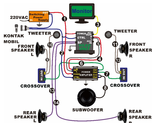
Gambar 9. Instalasi Sistem Audio Mobil dan titik trouble
