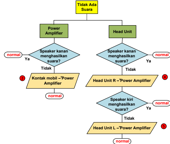
Gambar 11. Flowchart Saklar Trouble 2, 4 dan 5
