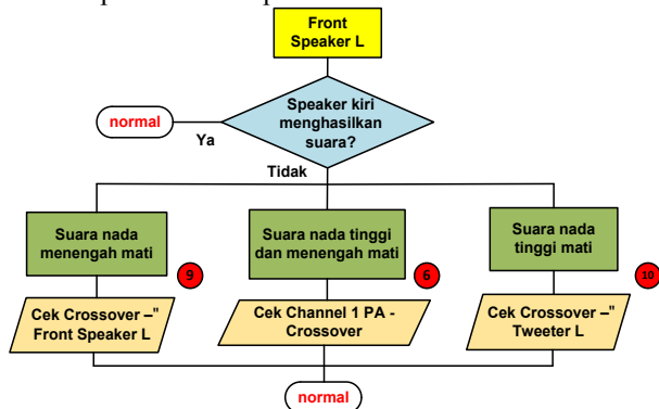
Gambar 12. Flowchart Saklar Trouble 6 dan 9
